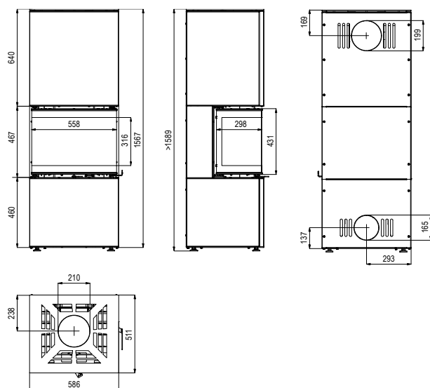
Rysunek 28. Wymiary wkładu kominkowego DEFRO HOME INTRA XSM C razem z zabudową w opcji COMPACT 1.
