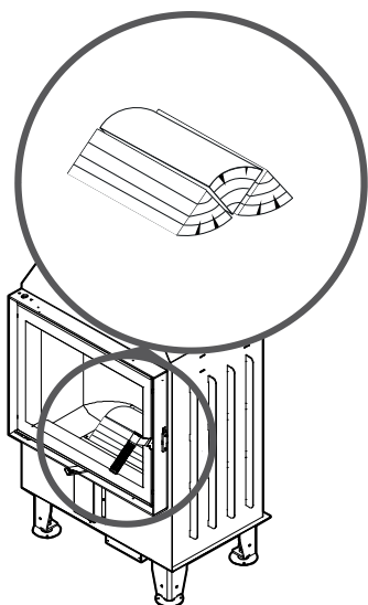
Rysunek 39. Sposób ułożenia paliwa
