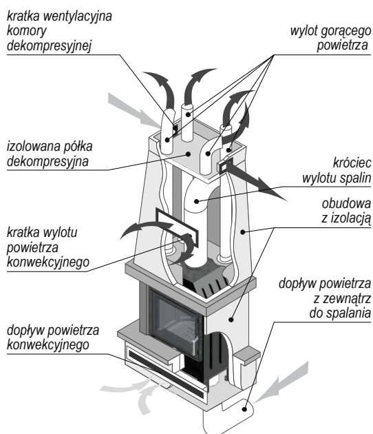
Rysunek 35. System dystrybucji gorącego powietrza.
