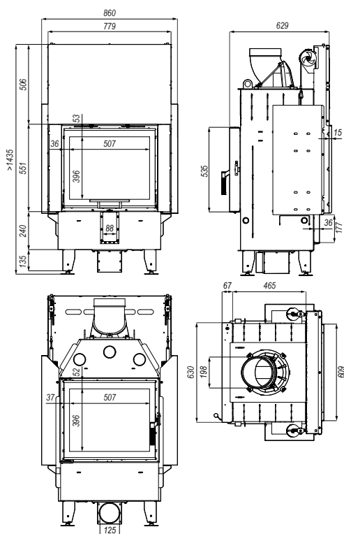
Rysunek 24. Wymiary wkładu kominkowego DEFRO HOME INTRA SM T G
