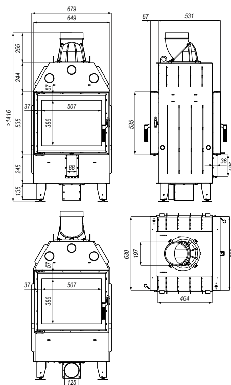
Rysunek 21. Wymiary wkładu kominkowego DEFRO HOME INTRA SM T.
