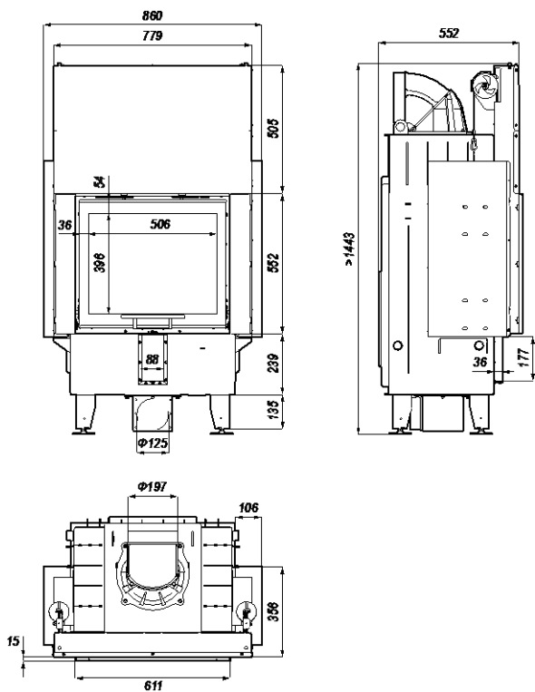
Rysunek 12. Wymiary wkładu kominkowego DEFRO HOME INTRA SM G
