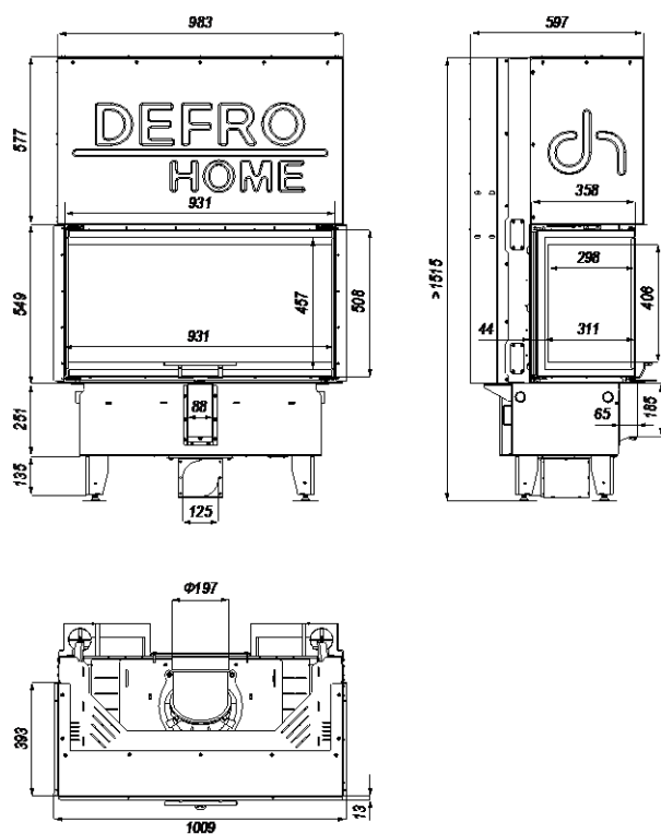
Rysunek 32. Wymiary wkładu kominkowego DEFRO HOME INTRA ME C G
