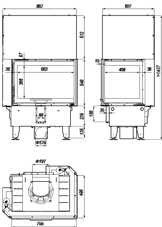
Rysunek 16. Wymiary wkładu kominkowego DEFRO HOME INTRA SM BP G.
