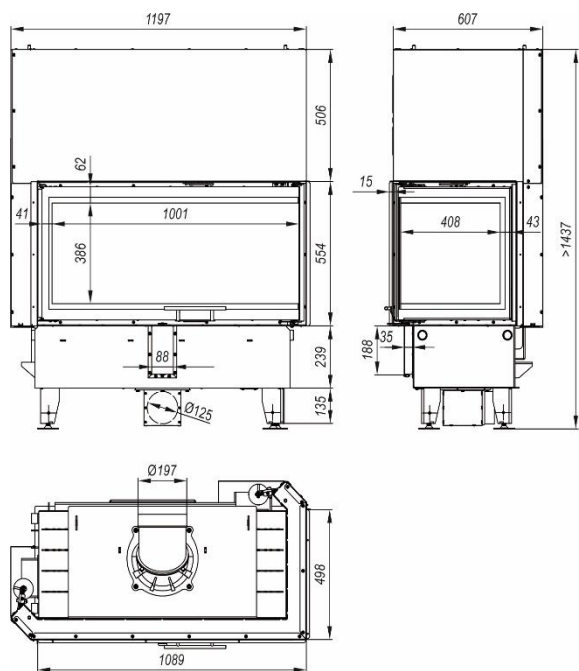
Rysunek 18. Wymiary wkładu kominkowego DEFRO HOME INTRA LA BP G
