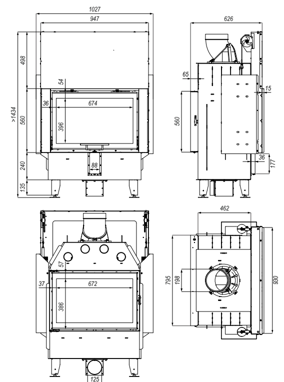
Rysunek 25. Wymiary wkładu kominkowego DEFRO HOME INTRA ME T G.
