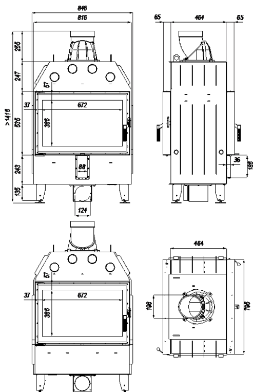
Rysunek 22. Wymiary wkładu kominkowego DEFRO HOME INTRA ME T.
