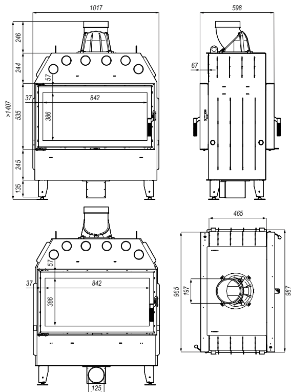
Rysunek 23. Wymiary wkładu kominkowego DEFRO HOME INTRA LA T
