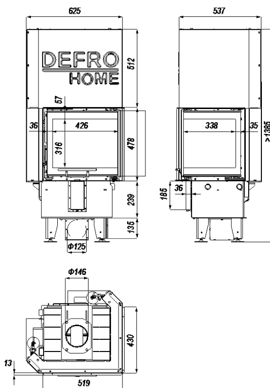
Rysunek 19. Wymiary wkładu kominkowego DEFRO HOME INTRA XSM BP MINI G.
