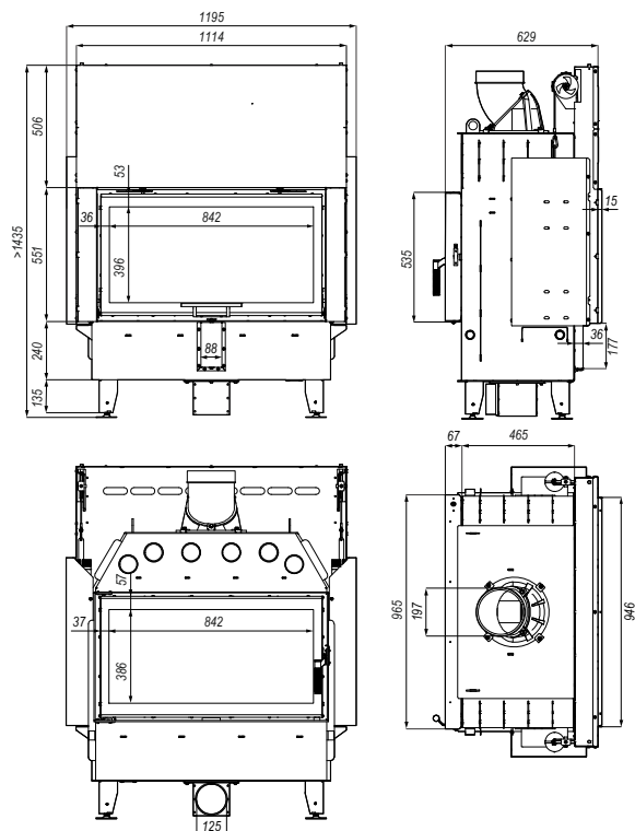
Rysunek 26. Wymiary wkładu kominkowego DEFRO HOME INTRA LA T G.
