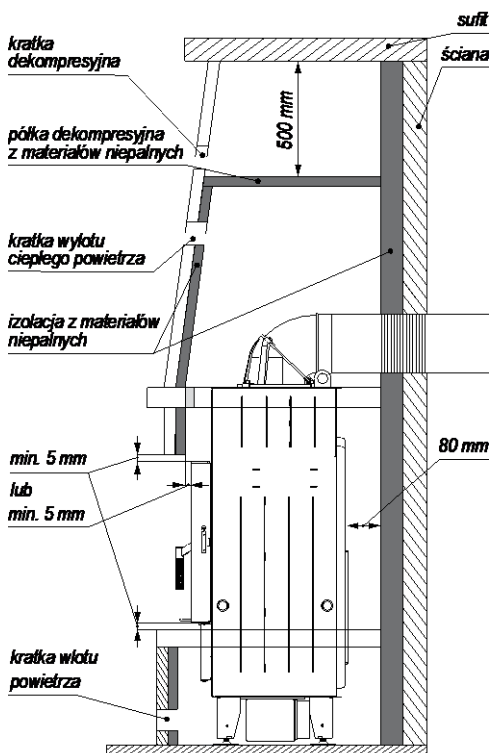
Rysunek 34. Przykładowa zabudowa wkładu kominkowego.
