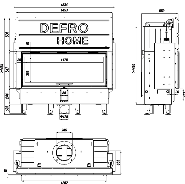
Rysunek 15. Wymiary wkładu kominkowego DEFRO HOME INTRA XLA G
