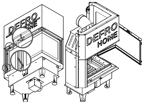
Rysunek 42. Umieszczenie rygli pozwalających na otwarcie drzwi w pozycji uchylnej z szybą boczną kominka DEFRO HOME INTRA w wersji BP(BL) G.
