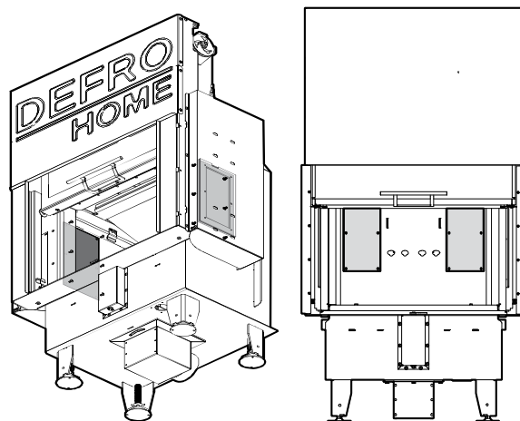
Rysunek 45. Umieszczenie pokryw otworów rewizyjnych we wkładach: DEFRO HOME INTRA wersji G (po lewej) i DEFRO HOME INTRA wersji C G (po prawej).
