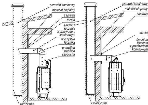
Rysunek 37. Podłączenie wkładu kominkowego do przewodu kominowego w zależności od wersji (po lewej wersji XSM i XLA, po prawej pozostałe).
