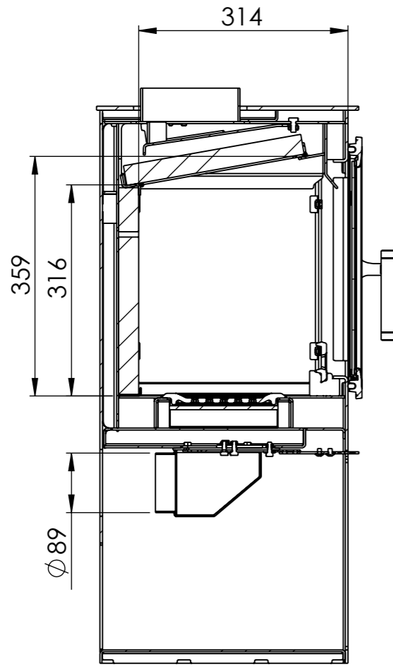
PRZEKRÓJ A-A SKALA 1 : 8
